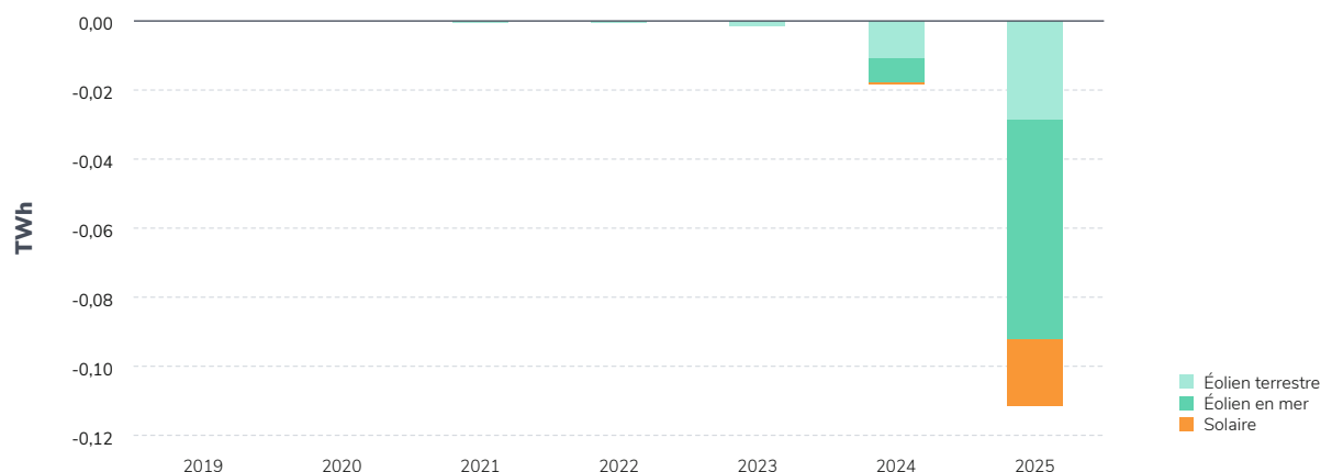
Figure 2.30 - Évolution des ajustements de production réalisés sur les filières éolienne et solaire
